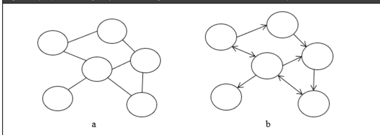
Figura 1. Ejemplo de a). Un grafo y b) una red dirigida, las flechas indican la dirección del flujo
